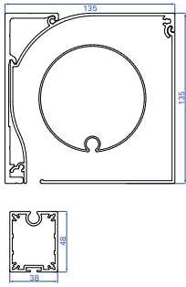
B1350
