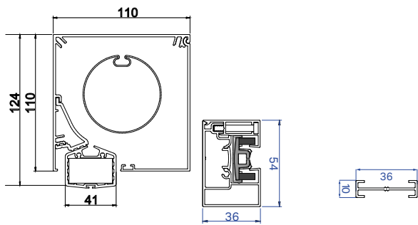
B1100 ZIP Prestige
